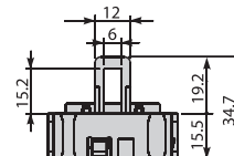
Modulo porta minifusibili Mini-fuses module 24.236.005
